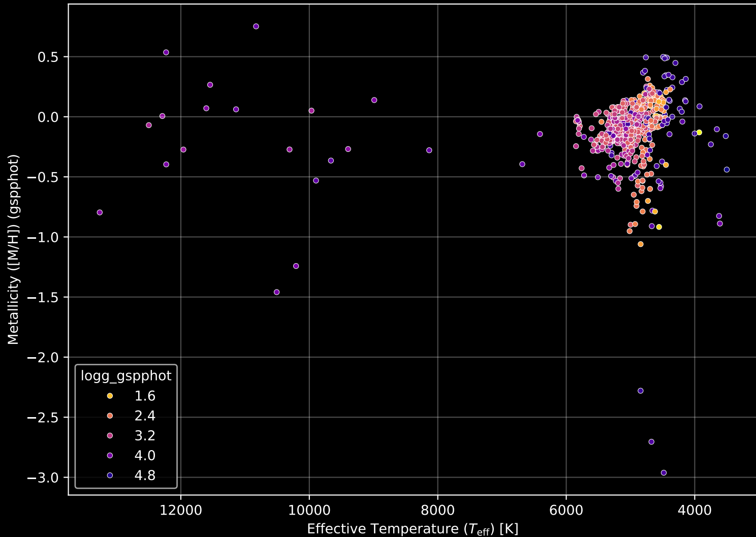
APOGEE DR17 Field: [150-08] Stellar Population Parameters (n= 564)
